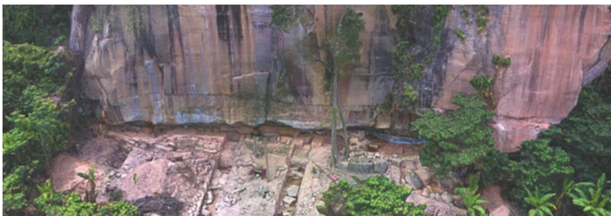
Localisation des sondages de l'abri sous roche de Poeng Ta Roet, vue de l'est.
